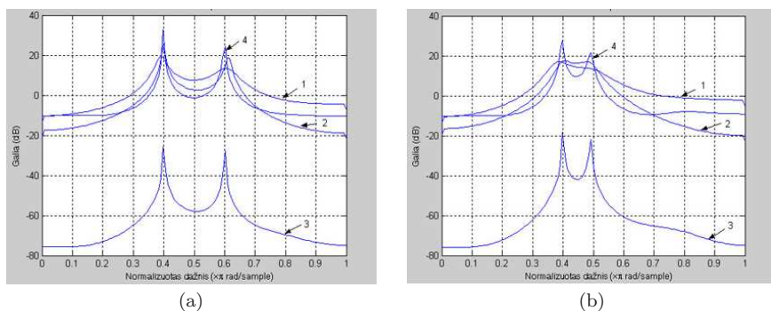
1 pav. Jule–Volkerio (1), Burgo (2), tikrinių reikšmių (3) ir MUSIC (4) metodų spekro įverčių palyginimas.
