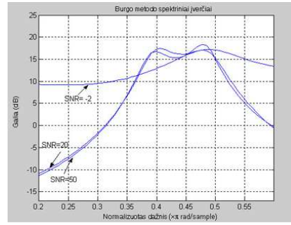
4 pav. Signalų spektriniai įvertiniai Burgo metodu.
