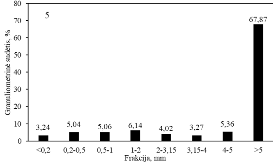
8 pav. Sugranuluoto kristalinio MAP granulimetrinė sudėtis, kai naudotas skirtingas 1 % koncentracijos krakmolo tirpalo kiekis: 1 – 5,0 %; 2 – 12,5 %; 3 – 17,5 %; 4 – 20,0 %; 5 – 25,0 %
