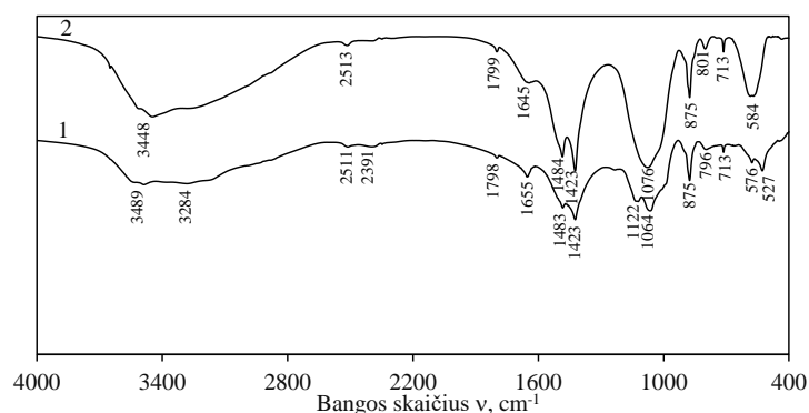
2 pav. \text{MgCO}_3 – \text{CaCO}_3 – \text{H}_3\text{PO}_4 – \text{NH}_4\text{F} – \text{H}_2\text{O} sistemoje gautų produktų FT-IR kreivė, kai izoterminio išlaikymo trukmė 80 °C (1) ir 120 °C (2) temperatūrose yra 8 h
